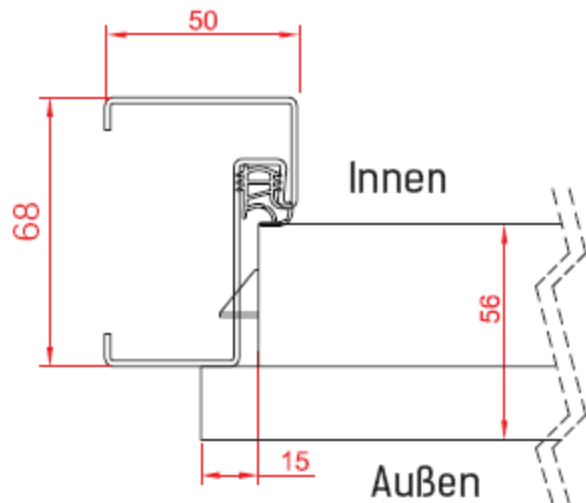
Querschnitt Tür
