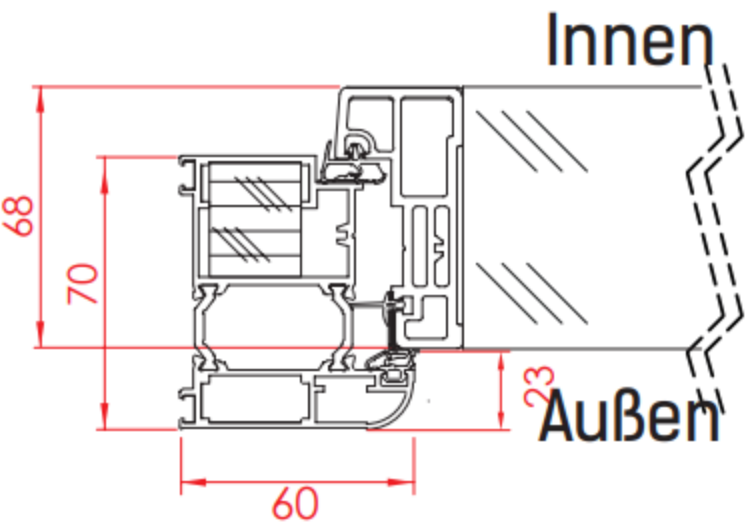
Rahmen Tür
