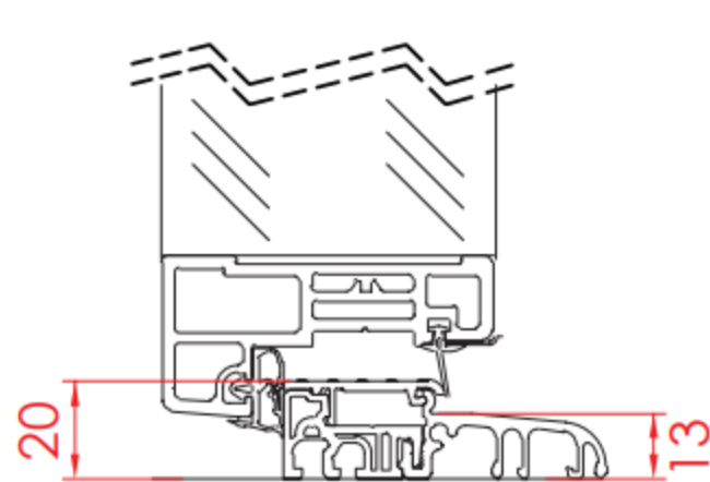
Schwelle
