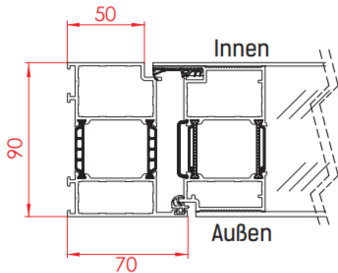
Querschnitt Tür
