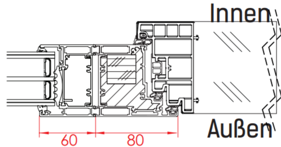
Seitenteil + Rahmen Tür
